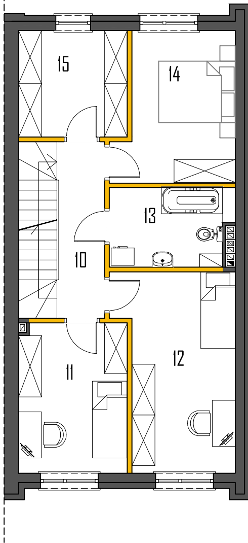
RZUT PIĘTRA
