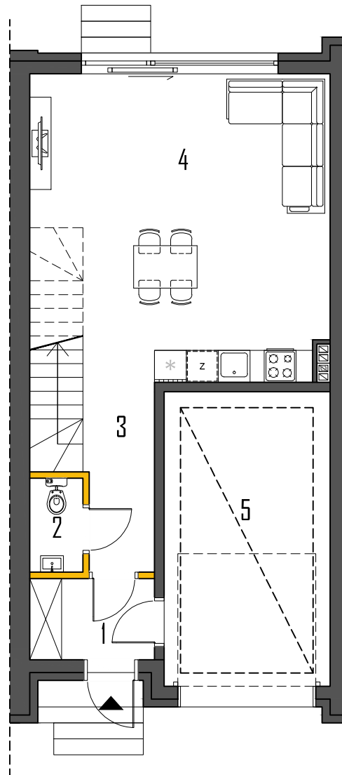
RZUT PARTERU
